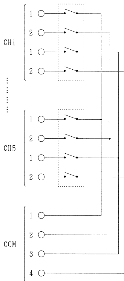
4線式選択時
