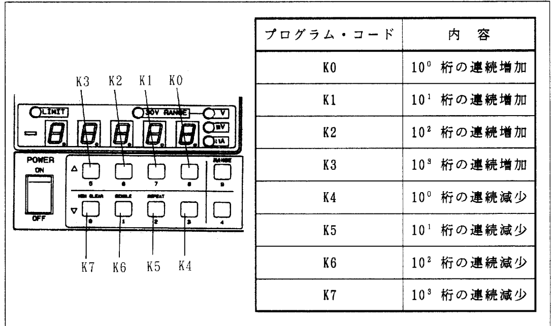
図 3 - 15 掃引動作と出力レベル桁
