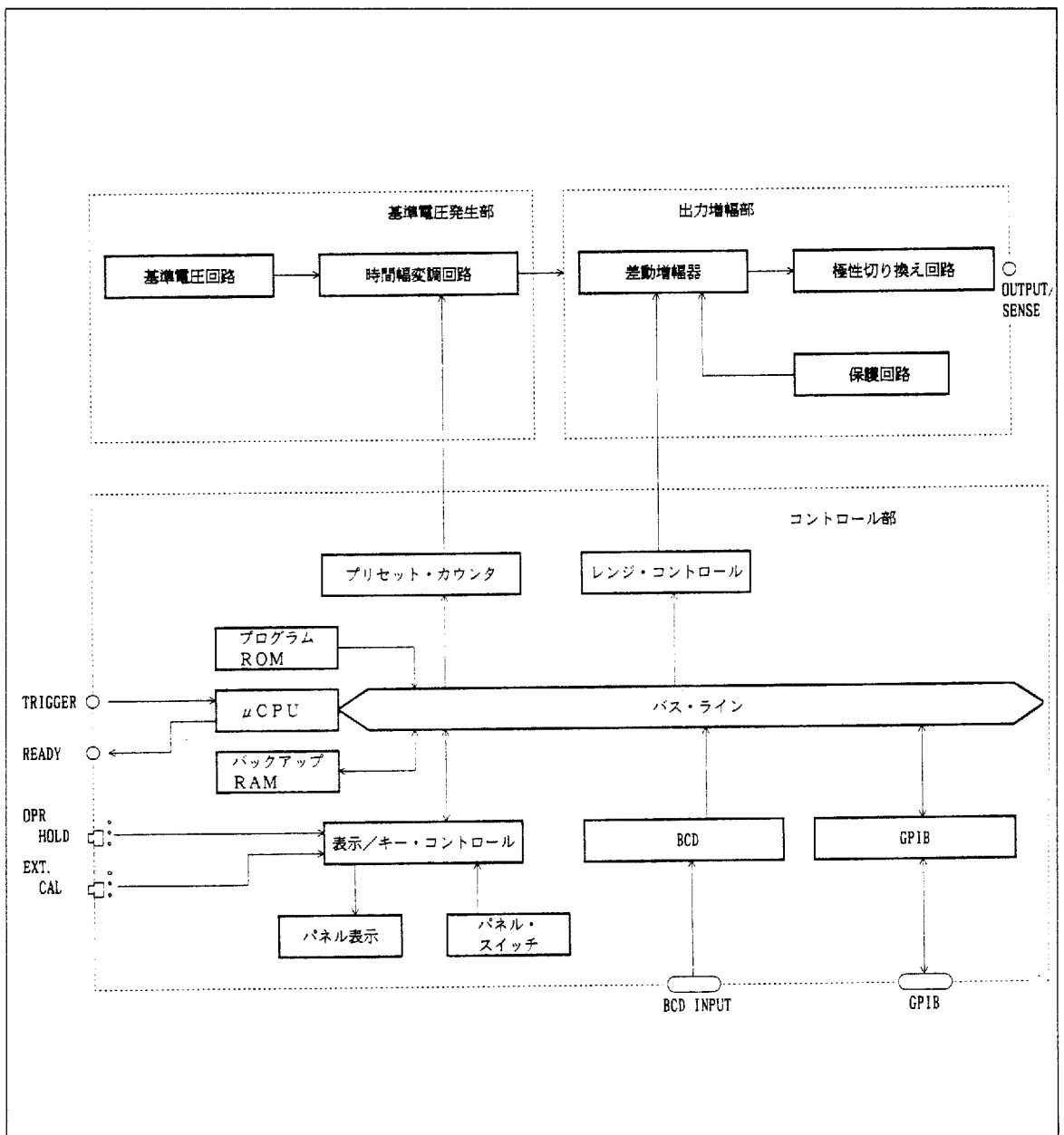
図 8 - 1 ブロック図
