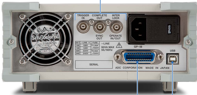
6240B リアパネル
